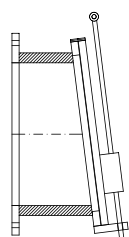
Zamknięcie awaryjne
